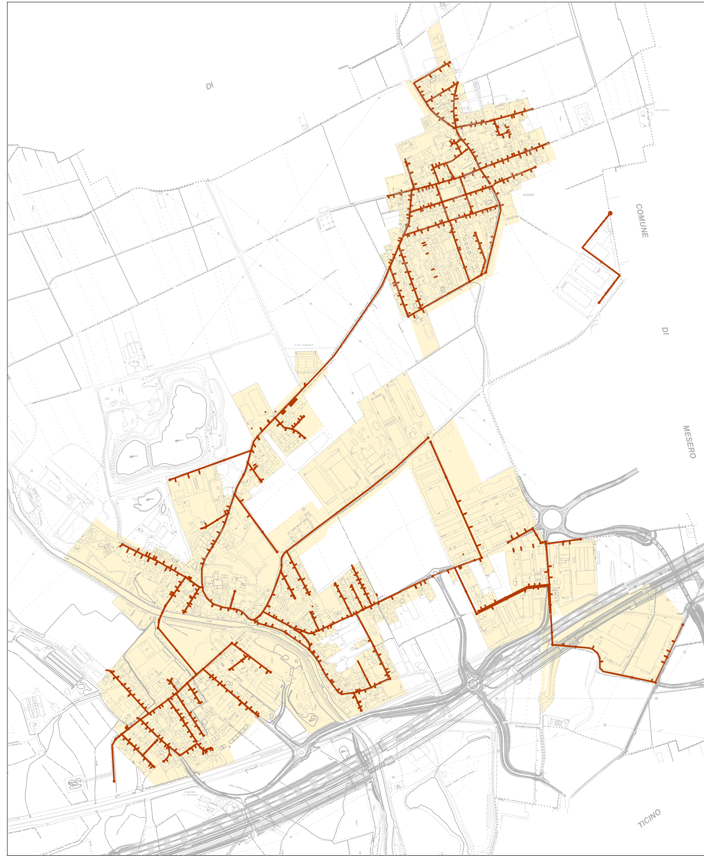
RETE DELLA FOGNATURA ESISTENTE
